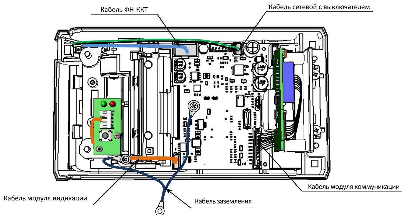
Рисунок 25. Расположение кабелей в нижней части корпуса АТОЛ 30Ф (БУ AL.P220.40.000 rev.1.1)
